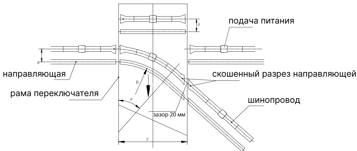
Плоский (параллельный) переключатель
